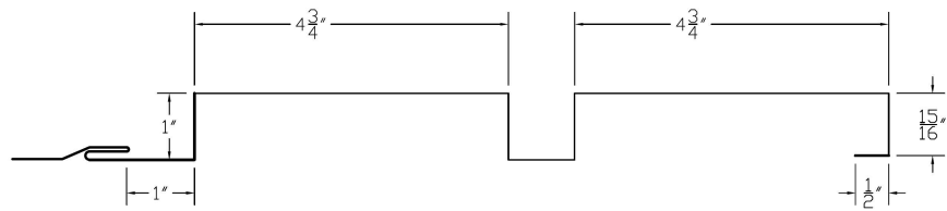
VariPanel™ 55.1 PLANK (SIDEVIEW)
