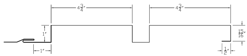
VariPanel™ 55.1 PLANK (SIDEVIEW)
