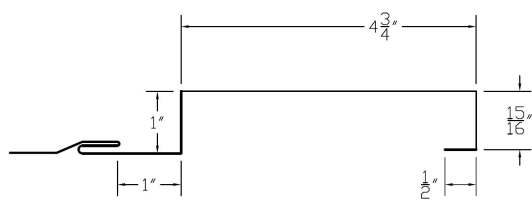
VariPanel™ 5.1 PLANK (SIDEVIEW)
